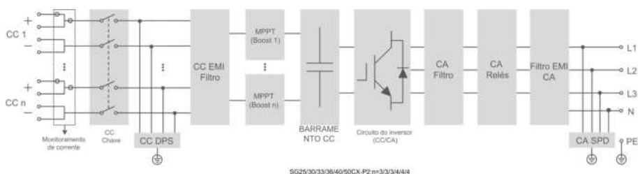
Figura 2-4 Diagrama do circuito
